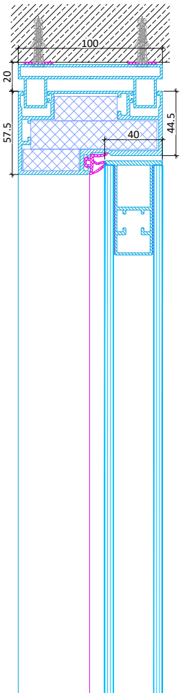
Alurahmentür Flush in raumhoher Zarge Vertikalschnitt
