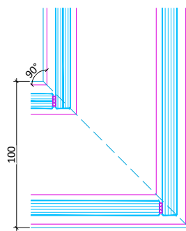
Holztür in raumhoher Zarge Vertikalschnitt
