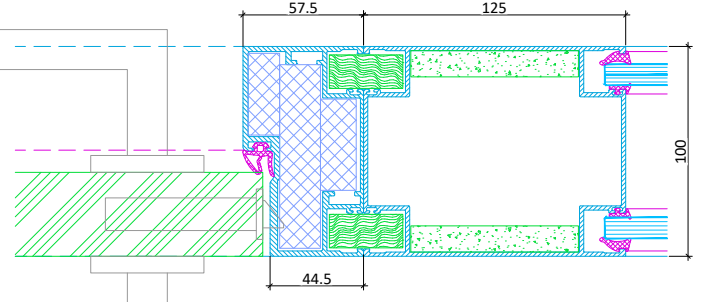
Holztür Schlossseite mit Türseitenteil Horizontalschnitt
