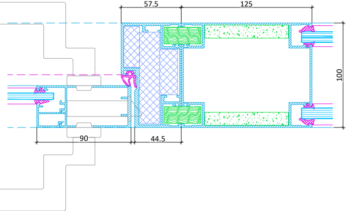
Alurahmentür Flush Schlossseite mit Türseitenteil Horizontalschnitt
