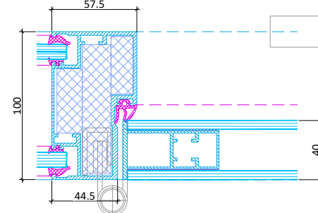
Alurahmentür Flush Bandseite Horizontalschnitt
