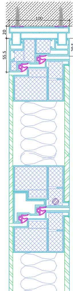
Vista DUO Volltür mit feststehender Oberblende Vertikalschnitt
