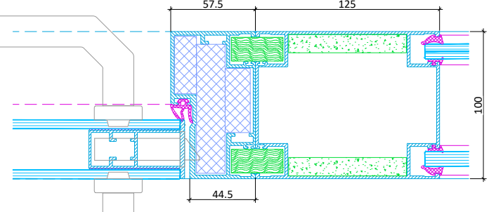
Alurahmentür Flush Schlossseite mit Türseitenteil Horizontalschnitt
