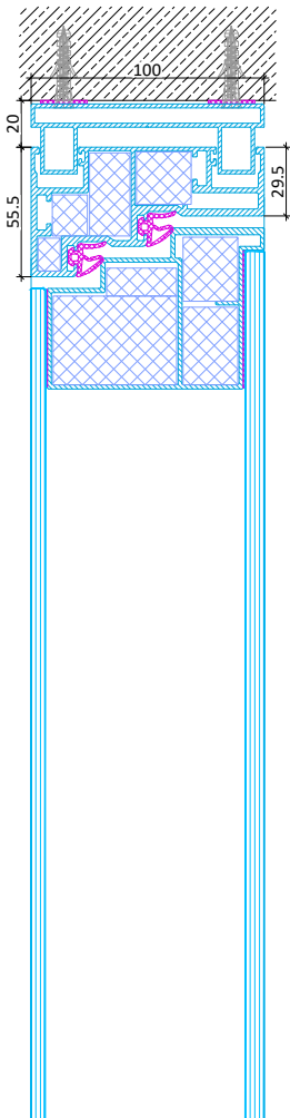
Vista DUO Glastür in raumhoher Zarge Vertikalschnitt
