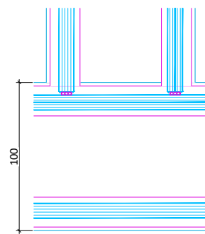
Alurahmentür Flush in raumhoher Zarge Vertikalschnitt
