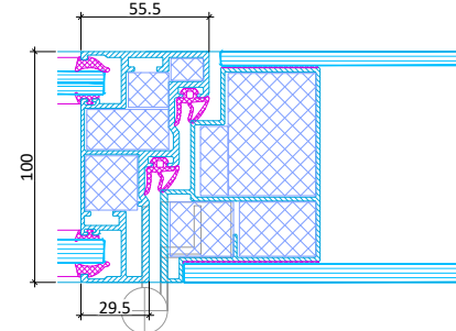
Vista DUO Glastür Bandseite Horizontalschnitt
