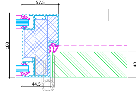
Holztür Bandseite Horizontalschnitt
