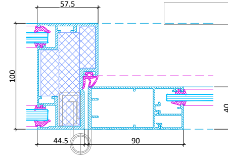
Alurahmentür Bandseite Horizontalschnitt
