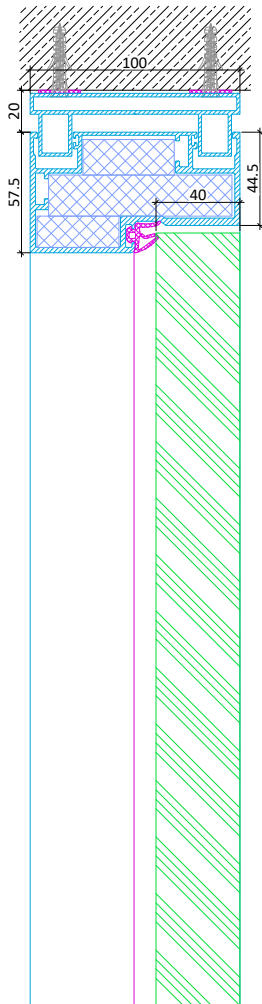
Holztür in raumhoher Zarge Vertikalschnitt
