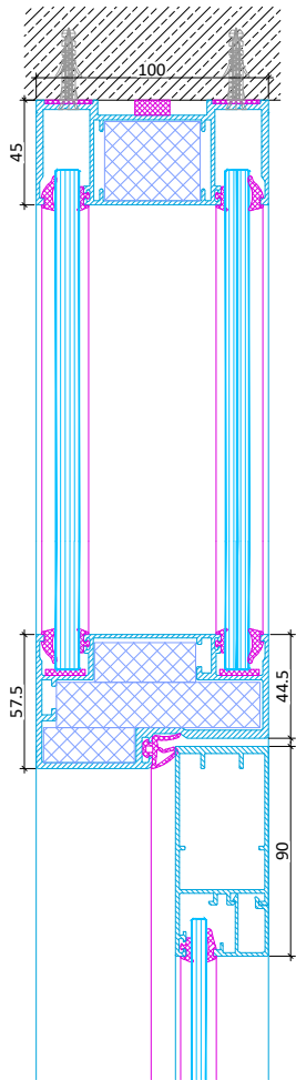
Alurahmentür mit Glasoberlicht Vertikalschnitt
