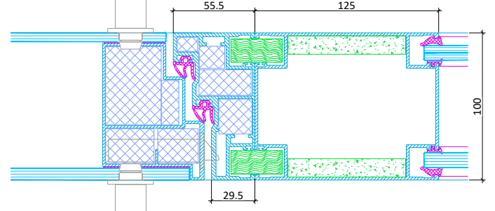
Vista DUO Glastür Schlossseite mit Türseitenteil Horizontalschnitt
