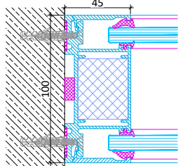
Verglasung Vertikalschnitt
