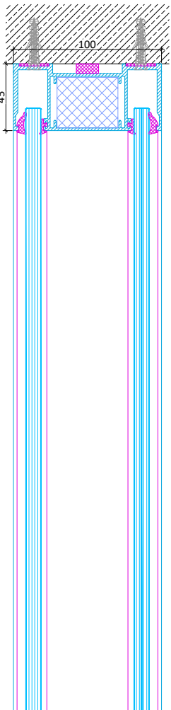
Verglasung Vertikalschnitt
