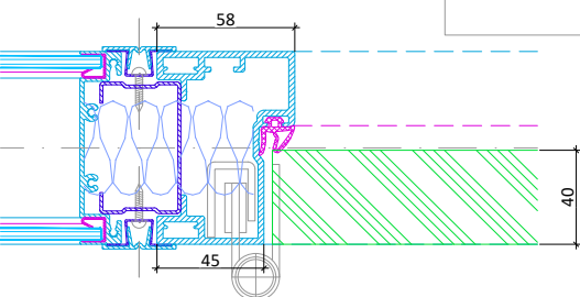
Holztür Bandseite Horizontalschnitt
