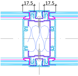
Ganzglastür mit Glasoberlicht Vertikalschnitt
