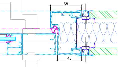
Alurahmentür Schlossseite mit Türseitenteil Horizontalschnitt
