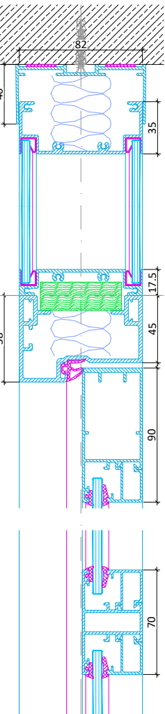
Alurahmentür mit Glasoberlicht Vertikalschnitt
