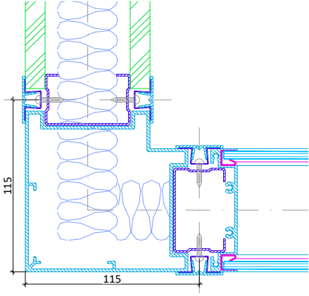
Holztür mit Glasoberlicht Vertikalschnitt
