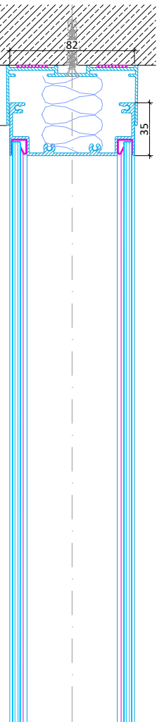
Ganzglaselement Vertikalschnitt
