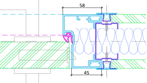
Holztür Schlossseite mit Türseitenteil Horizontalschnitt
