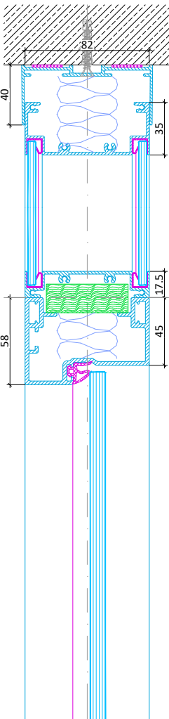
Ganzglastür mit Glasoberlicht Vertikalschnitt
