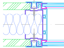
Ganzglaselement Vertikalschnitt
