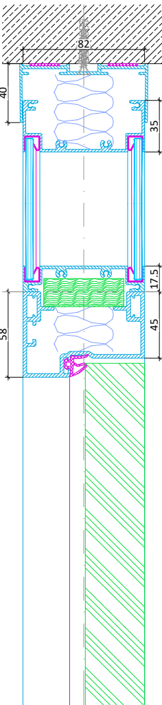
Holztür mit Glasoberlicht Vertikalschnitt
