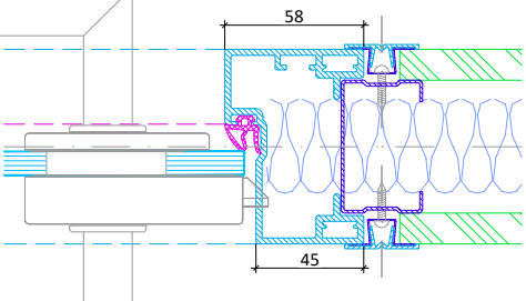
Ganzglastür Schlossseite mit Türseitenteil Horizontalschnitt
