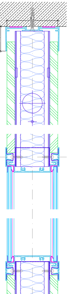
Brüstungsfenster Vertikalschnitt
