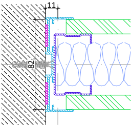
Beplankung Vertikalschnitt
