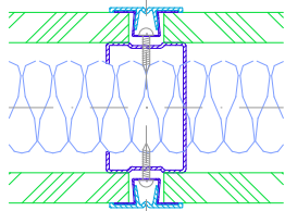
Brüstungsfenster Vertikalschnitt
