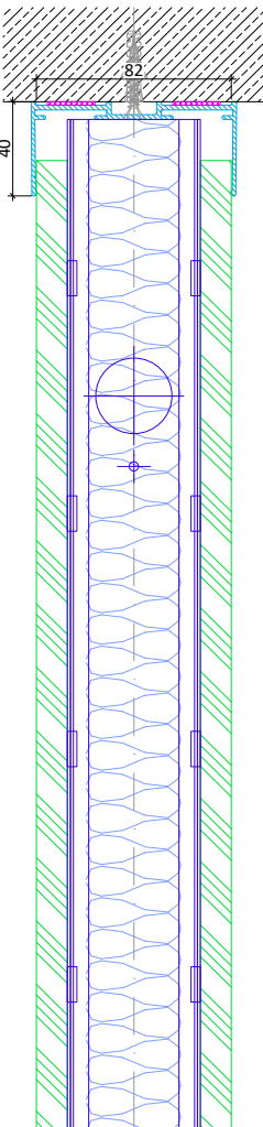
Beplankung Vertikalschnitt
