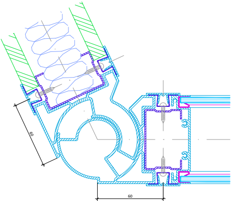
Variabler Eckpfosten Horizontalschnitt
