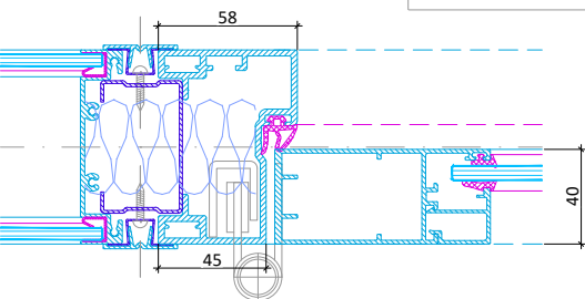
Alurahmentür Bandseite Horizontalschnitt
