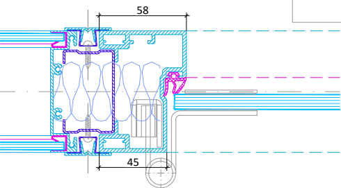
Ganzglastür Bandseite Horizontalschnitt
