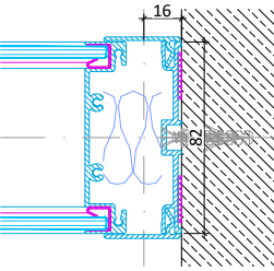
Alurahmentür mit Glasoberlicht Vertikalschnitt
