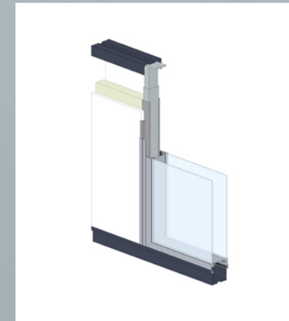
Lehnertwand Industrie, mit innenliegender Rohrstütze und Teleskop-Deckenanschluss
