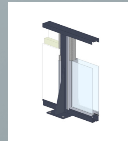
Lehnertwand Industrie, freistehend mit Fußplatte und Knappe ab Wandhöhe 3.000 bis max. 3.500 mm
