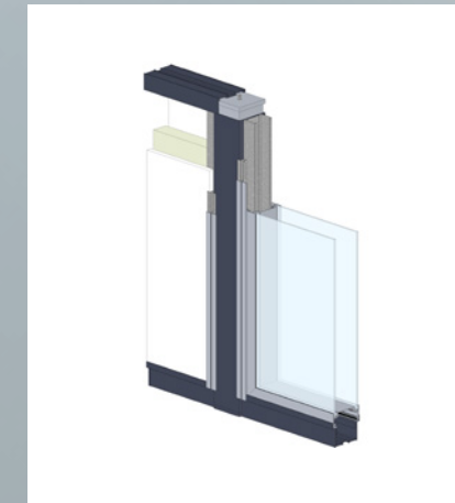
Lehnertwand Industrie, mit sichtbarer Rohrstütze und Teleskop-Deckenanschluss
