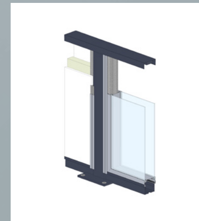
Lehnertwand Industrie, freistehend mit Fußplatte bis Wandhöhe 3.000 mm
